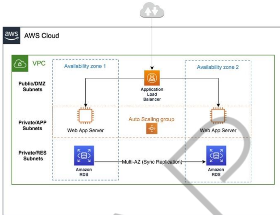
Figura 1 – VPC Fonte: AWS (2025)
